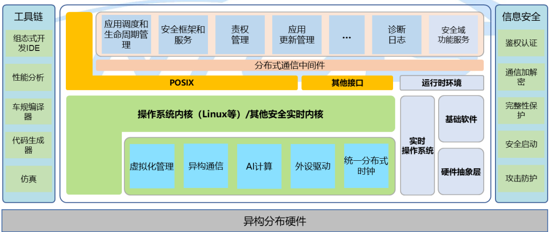
图 16 系统软件架构
