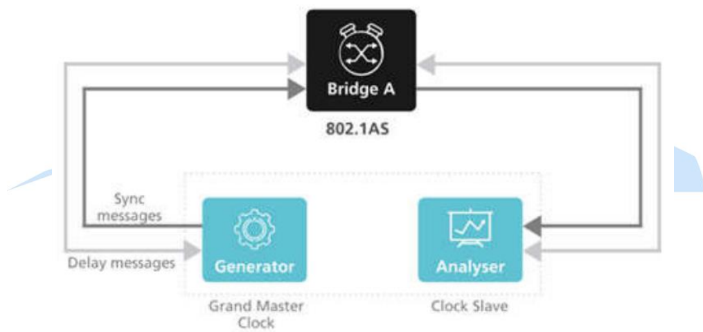
图 18 TSN 时间同步基本流程
