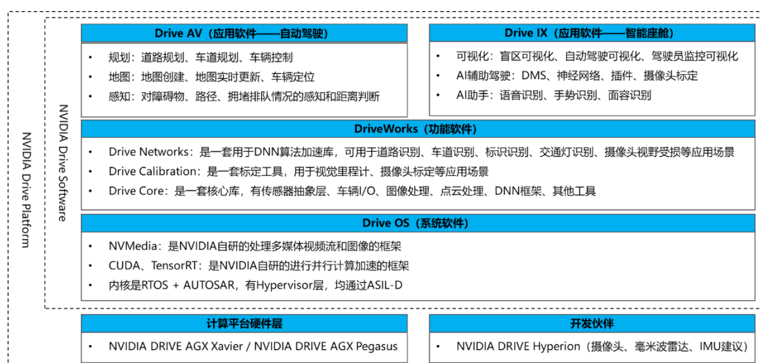
图 13 英伟达自动驾驶平台架构
