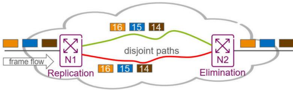
图 20 TSN 可靠性工作原理
