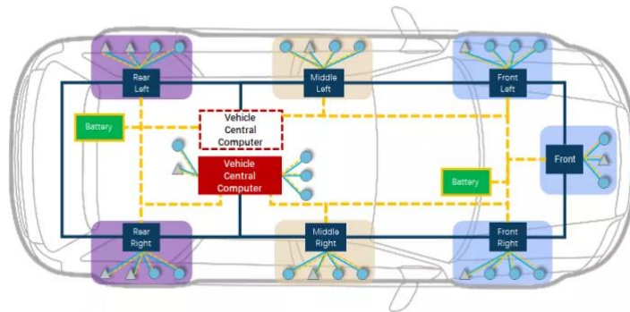
图 4 Zonal EEA 示意图（来源于网络）
