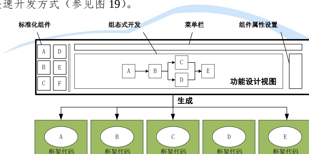
图 19 组态式开发 IDE 框架
