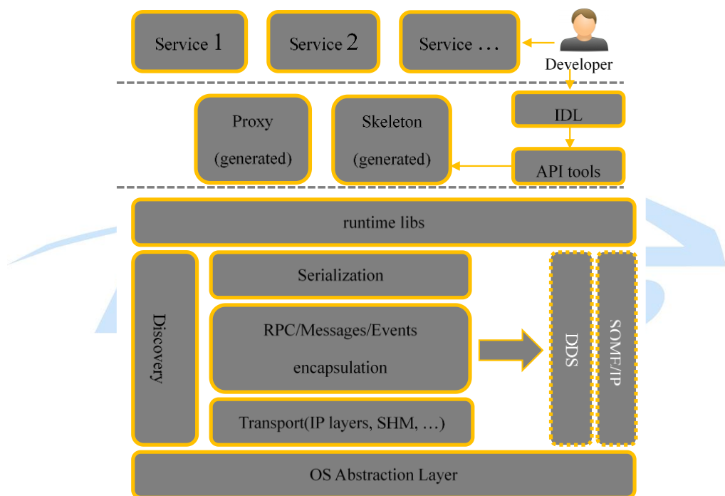
图 17 分布式通信中间件 SOA 架构
